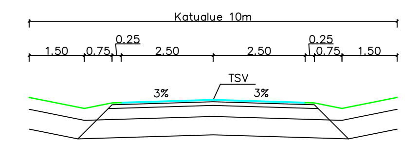
POIKKILEIKKAUS 1:100
