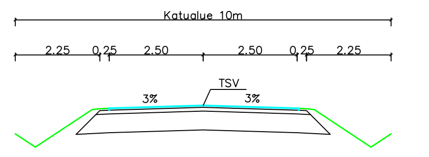
POIKKILEIKKAUS 1:100 PL 40-396
