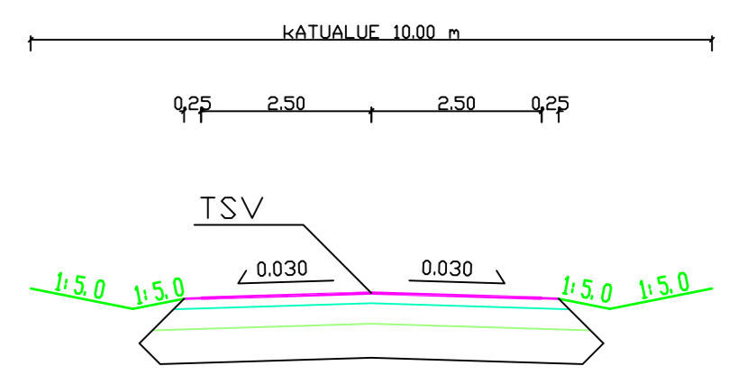
POIKKILEIKKAUS 1:100
