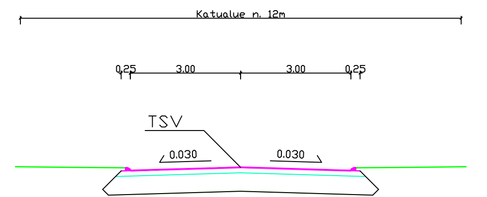
POIKKILEIKKAUS 1: 100
